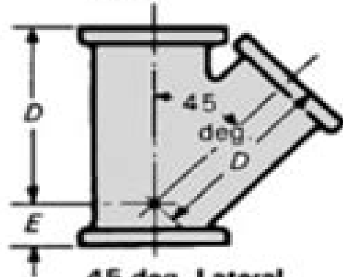
45 deg. Lateral
