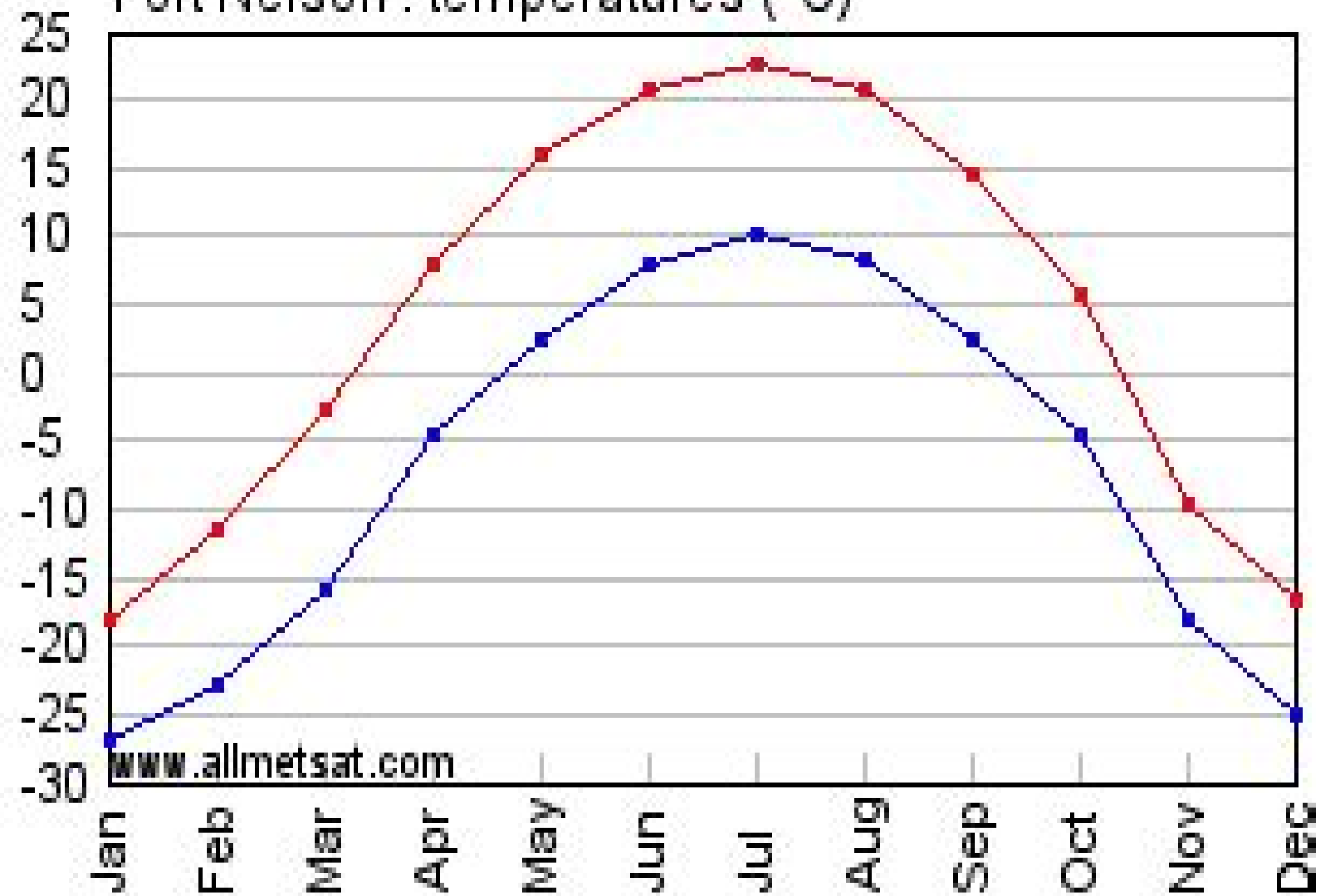
Fort Nelson : temperatures (°C)
