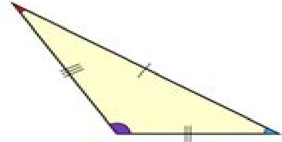
Scalene
