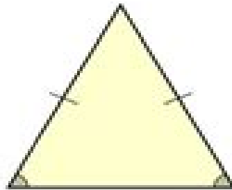
Isosceles
