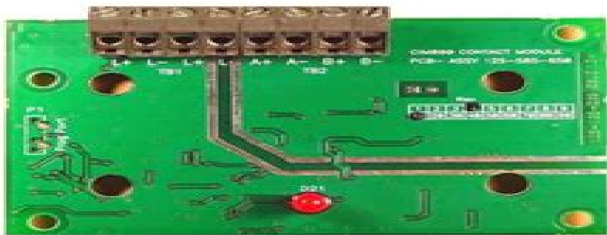
Fig. 1: CIM800 Contact Input Module
