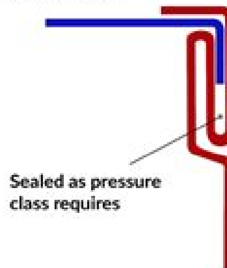
Hammer Over Edge
