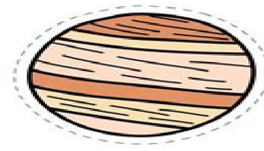
Jupiter
