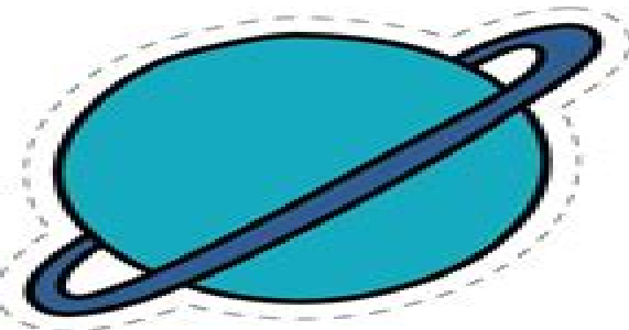
Uranus
